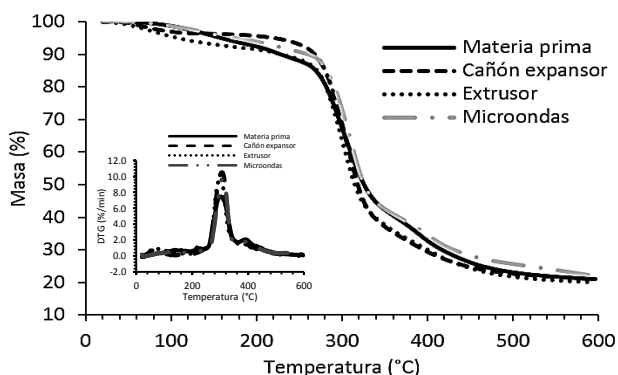
Figura 3.4. TG y DTG de materia prima e insuflados de quinua sin recubrimiento. Fuente: elaboración propia.
