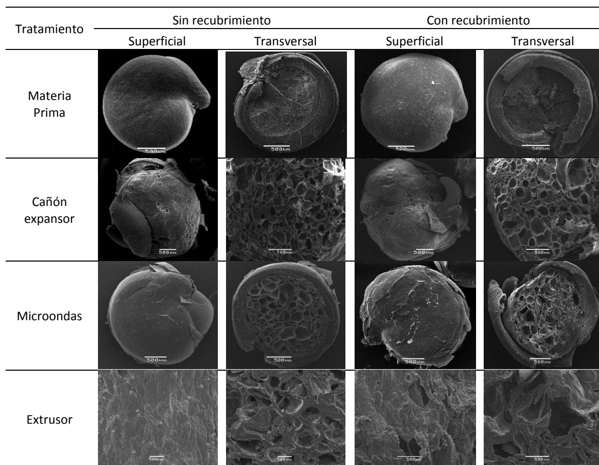
Figura 3.3. Microestructura de insuflados de quinua, Roja INIA, con y sin recubrimiento, procesadas mediante tres tratamientos térmicos. Fuente: elaboración propia.
