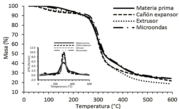
Figura 3.5. TG y DTG de materia prima e insuflados de quinua con recubrimiento. Fuente: elaboración propia.
