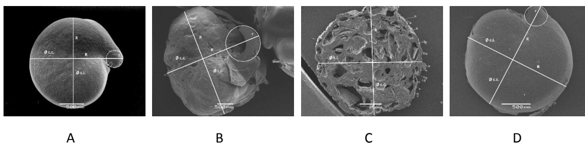
Figura 3.1. Mediciones de microfotografías de granos de quinua: (A) materia prima, (B) cañón expansor, (C) extrusor y (D) microondas. Fuente: elaboración propia.
