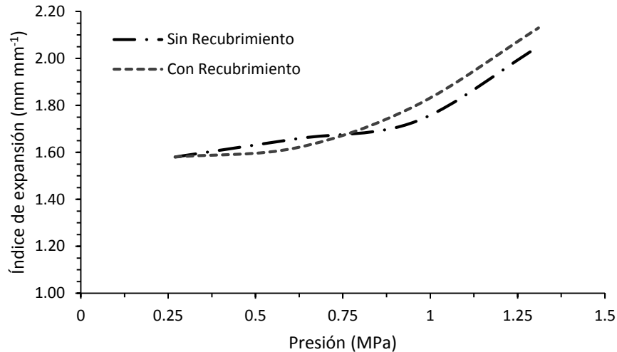
Figura 2.3. Expansión de granos de quinua con y sin recubrimiento a 20 % de humedad (bh) tratados mediante cañón expansor en función de la presión de operación. Fuente: elaboración propia.
