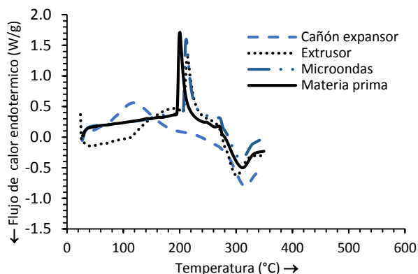
Figura 3.6. DSC de materia prima e insuflados de quinua sin recubrimiento. Fuente: elaboración propia.
